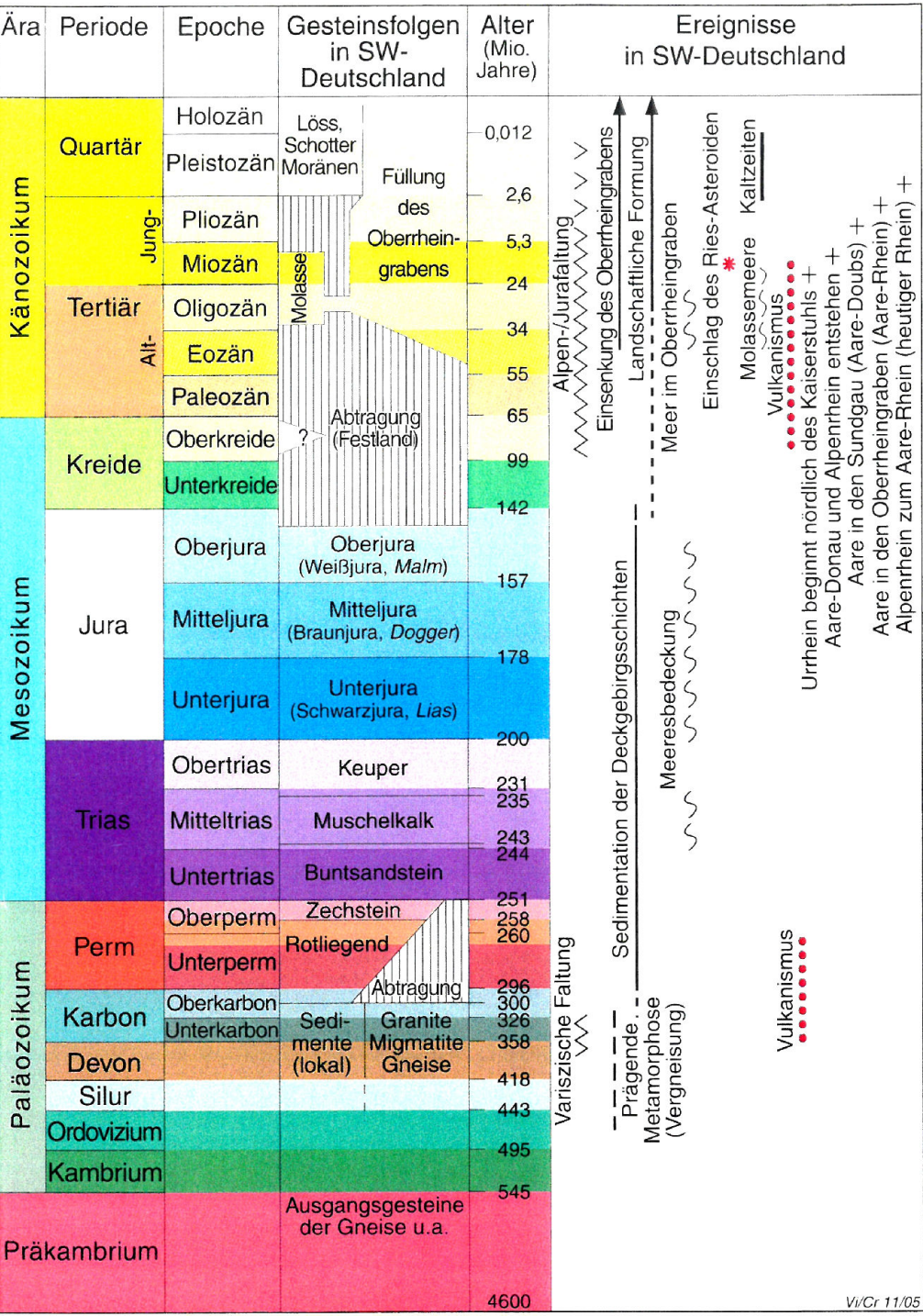
Endgeschichtliche Gliederung und Ereignisse in Süddeutschland, nach GROSCHOPF & VILINGER (1998, ergänzt). - Grafik: LGRB.
